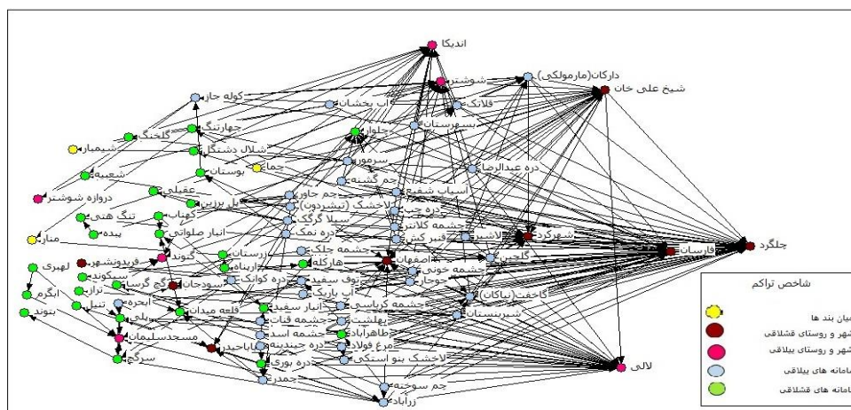
شکل ۶. دیاگرام تراکم
