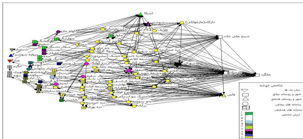
شکل ۹. دیاگرام خوشه‌ای
